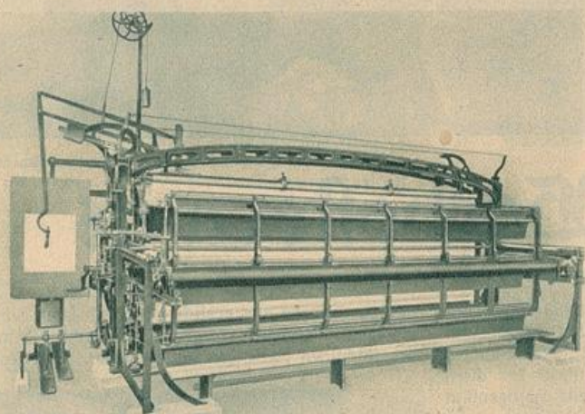
Dreistöckige Handstickmaschine der Vogtländischen Maschinenfabrik A. G., Plauen. Modell um 1908.
