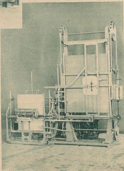
Punchmaschine mit Kontrollstickmaschine (Vorderansicht).
